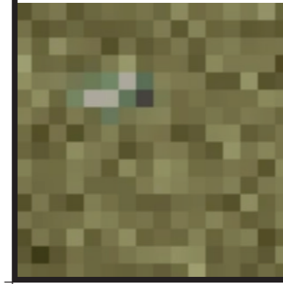
SKARN
