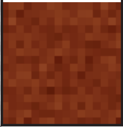
BOKSIT
