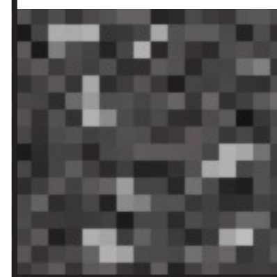
GABBRO
